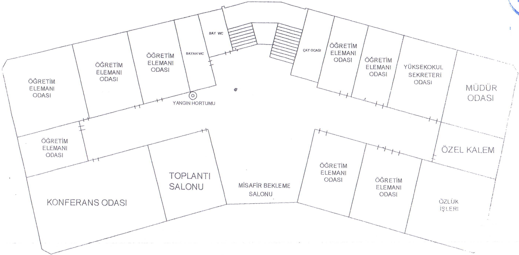
1. KAT PLANI_A BLOK
